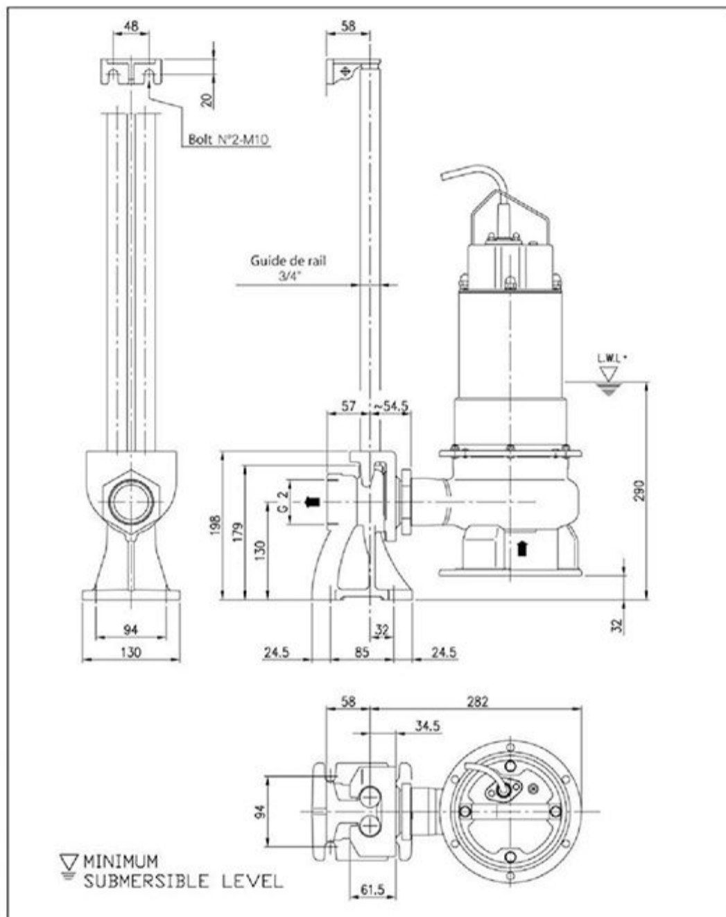
ابعاد كيت كوپلنگ DW-DW VOX
