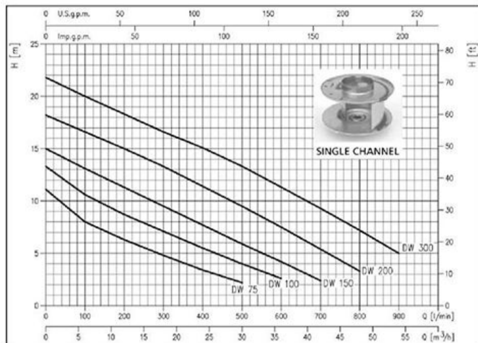
منحنی های راندمان DW
