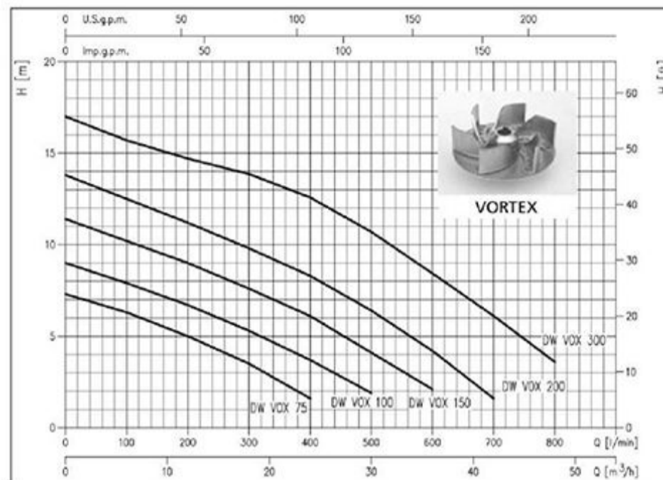
منحنی های راندمان DW VOX
