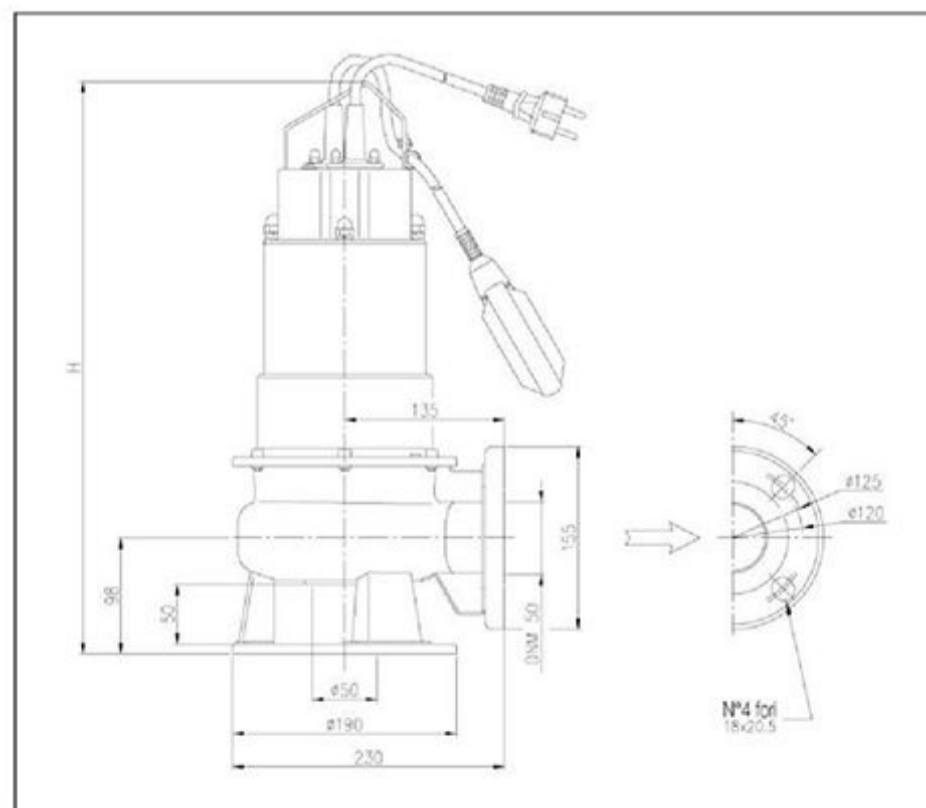
ابعاد DWF-DWF VOX
